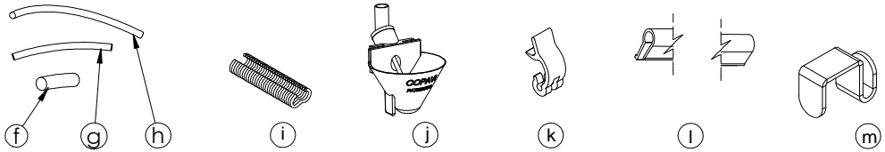
(f) COD. 75212100 Tubo pvc 6 cm 6x (g) COD. 75212600 Tubo pvc 38 cm 2x (g1) COD. 75213200 Tubo pvc 48 cm 3x (g2) COD. 75213000 Tubo pvc 21 cm 2x (h) COD. 75213200 Tubo pvc 125 cm 1x COD. 03035400 Grapas COD. 03034200 Bebedero copavi 6x COD. 01050100 Cierre plástico 6x COD. 73512100 Junquillo plást. rojo 2x COD. 73070301 Enganche cesta 8x
