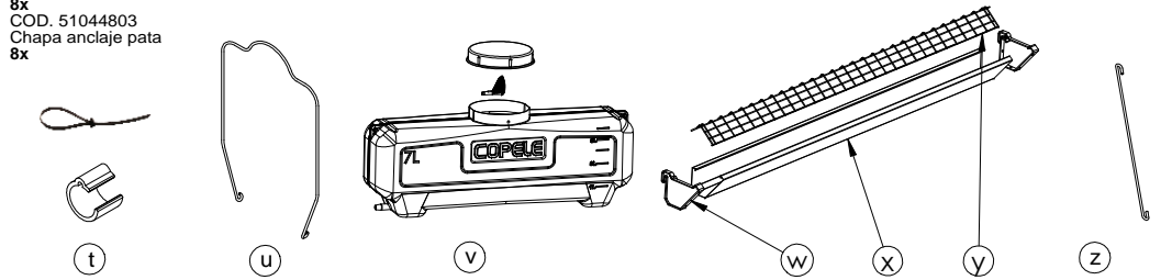
COD. 77013700 Torn. DIN 933 M6x35 8x COD. 01047600 Tuerca DIN 934 M6 8x COD. 03082700 Arandela M6 ala ancha 8x COD. 51044803 Chapa anclaje pata 8x COD. 01026400 Derivacion T 5x COD. 01037300 Codo plastico 3x COD. 03041900 Taconera de plástico 8x COD. 03073200 Pata arco 2x COD. 03073300 Pata arco 2x COD. 53070702 Anclaje pata COD. 53070702 Anclaje pata COD. 77013700 Torn. DIN 933 M6x35 8x COD. 01047600 Tuerca DIN 934 M6 8x COD. 03082700 Arandela M6 ala ancha 8x COD. 51044803 Chapa anclaje pata 8x COD. 01026400 Derivacion T 5x COD. 01037300 Codo plastico 3x COD. 03041900 Taconera de plástico 8x COD. 03073200 Pata arco 2x COD. 03073300 Pata arco 2x COD. 53070702 Anclaje pata COD. 53070702 Anclaje pata COD. 75213300 Gancho tope huevo 8x (x) COD. 53070601 Canal base prelacado 2x (y) COD. 03072600 Rejilla anti-desp. Rectangular 2x (W) COD. 03072000 Boquilla plástico dcha. comedero 2x COD. 03073000 Boquilla plástico izda. comedero 2x
